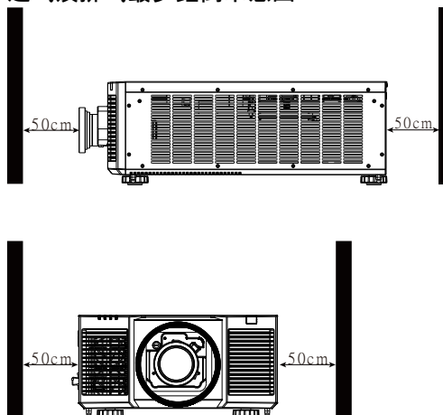
进气及排气最少距离示意图
