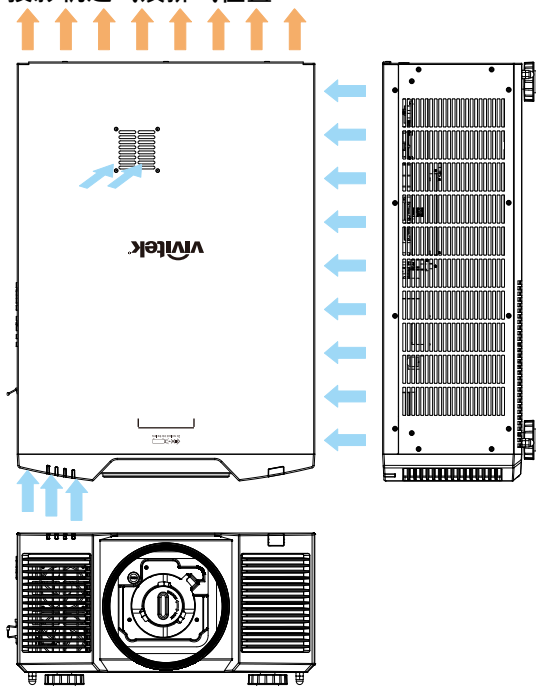
投影机进气及排气位置
