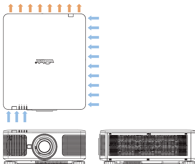
Поток воздуха и теплоотдача
