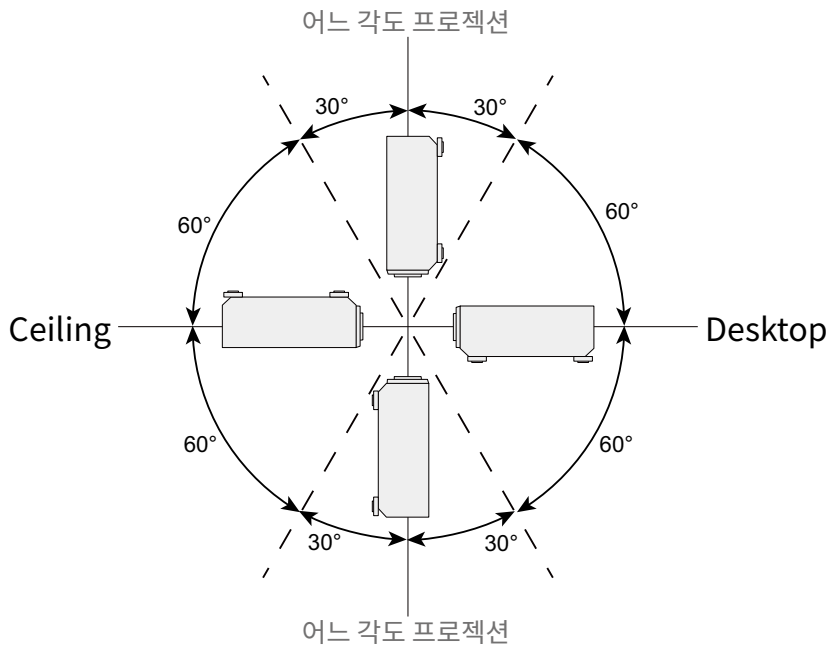
식탁, 천장 과 어느 각도 프로젝션 설치
