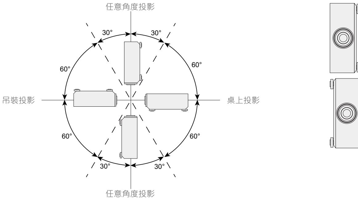
桌上安裝、吊裝及任意角度安裝
